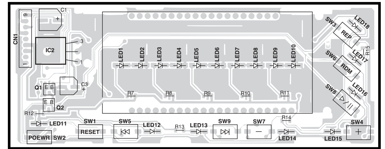
DISPLAY UNIT
